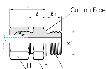
Form B stud end
